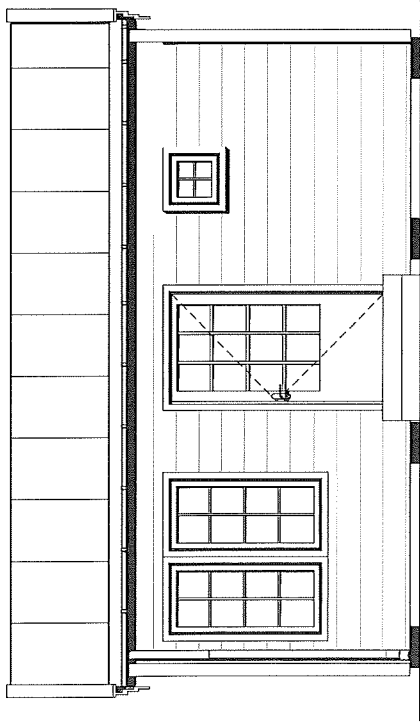
Fasad mot öst
